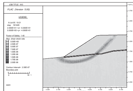
Rys. 3. Mapa przyrostów odkształceń postaciowych dla wariantu W3
