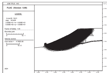
Rys. 4. Wektory prędkości dla wariantu W3
