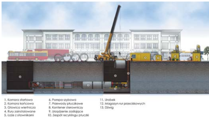
Ryc. 5. Przykład technologii bezwykopowej
