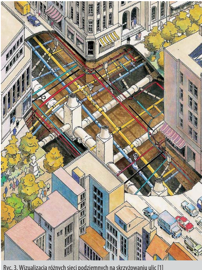
Ryc. 3. Wizualizacja różnych sieci podziemnych na skrzyżowaniu ulic [1]
