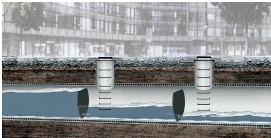
Wizualizacja retencyjnego kanału ściekowego, Uponor Infra Sp. z o.o.
