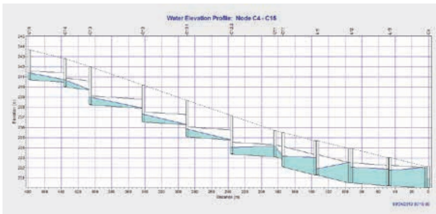
Profil hydrodynamiczny kanału retencyjnego, Politechnika Rzeszowska
