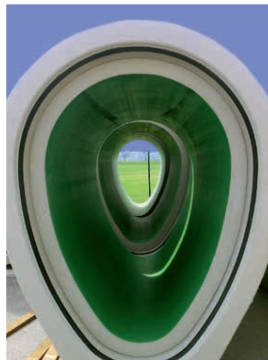
Rura o profilu jajowym z okładziną PEHD, fot. HABA-Beton Johann Bartlechner Sp. z o.o.
