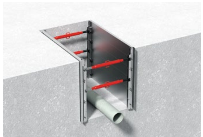
System liniowy LITEBOX
